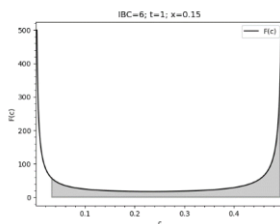
Рис. 2. Визуализация расчета интеграла для положения x = 0.15
