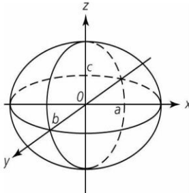
Рис 1. Эллипсоид.
