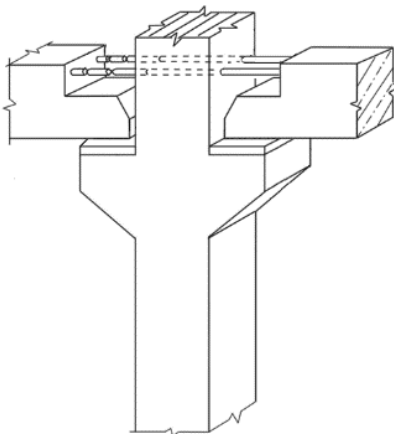
Рис. 2 Соединение ригеля с колонной
