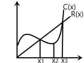
Рис.2. Нахождение прибыли при нелинейной функции издержек
