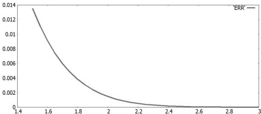
Рис.1. График оценки ошибки
