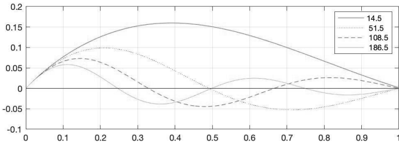
Рис. 1. График собственных функций задачи (8) – (9) при a = 1, b = 2 и \alpha = 1.3
